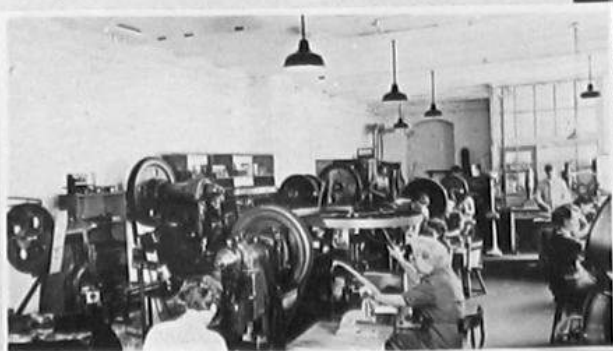
Stanzerlei im Hintergrund Spritzlackieren Stamping shop- spray varnishing
